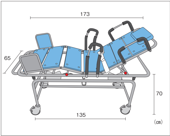
寝位入浴(分離式ストレッチャーでの入浴)
